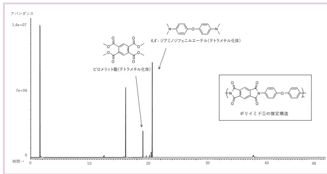
図2-1 ポリイミド①の超臨界メタノール分解GC-MSクロマトグラム
