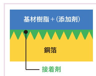
図1 プリント配線板の断面概要図
