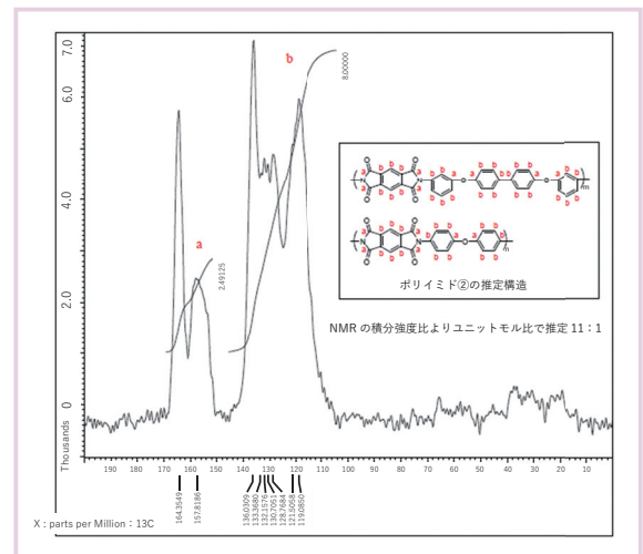
図2-3 ポリイミド②の固体 13 C-NMRスペクトル
