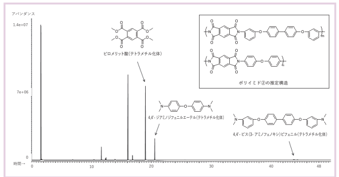
図2-2 ポリイミド②の超臨界メタノール分解GC-MSクロマトグラム
